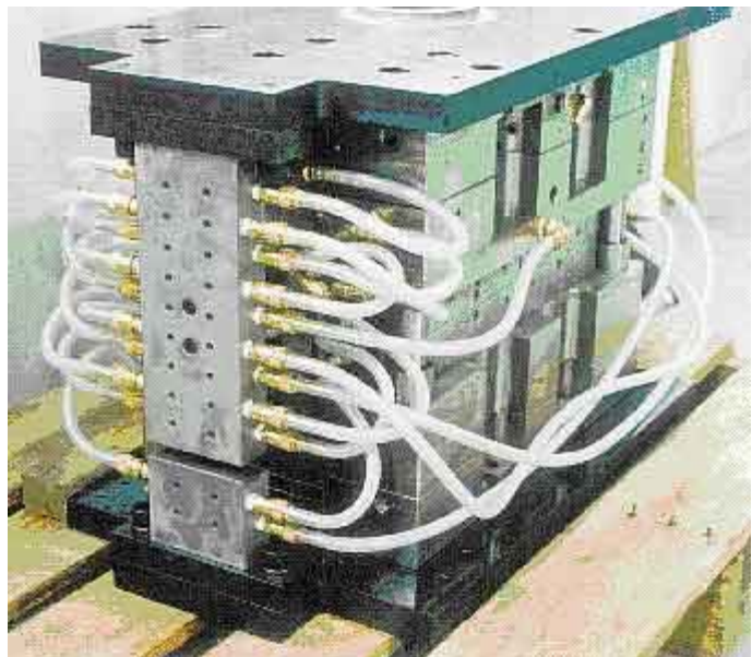
金型側（面シールタイプ）
