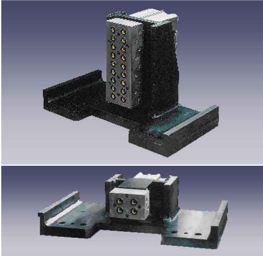
金型側（面シールタイプ）
